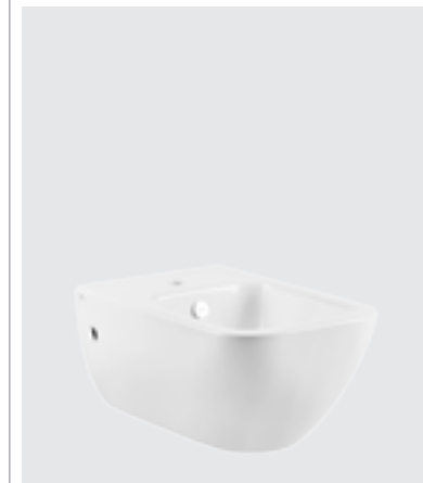
355x 540 x 272/420 h mm 39115
